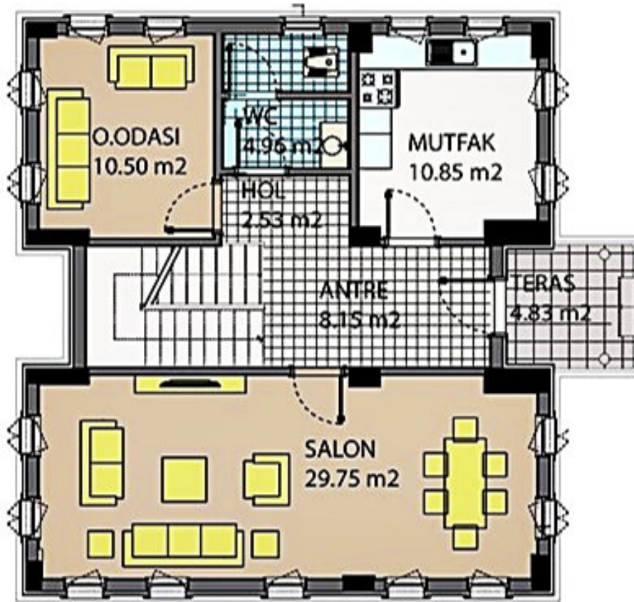
ZEMİN KAT PLANI
